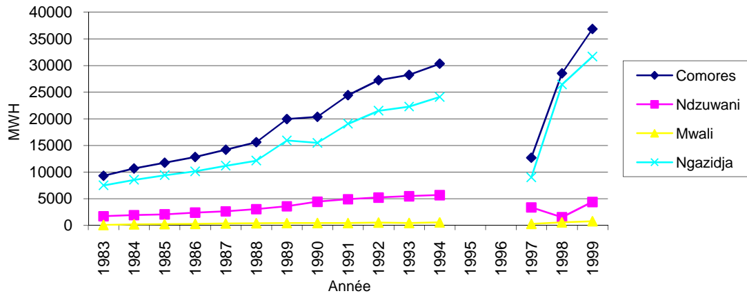
Figure 1 : Evolution de la production d'électricité
